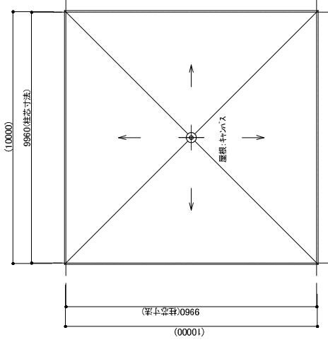
屋根伏図 1/150
