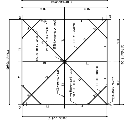
小屋伏図 1/150
