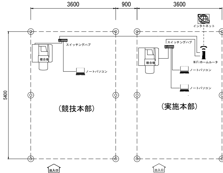
ネットワーク図 パイプメント1.5K×2K(天幕:白)×1
