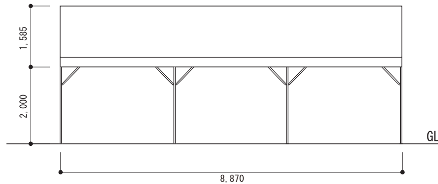
側面図
