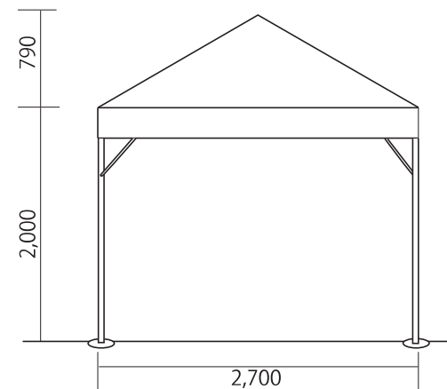
立面図
