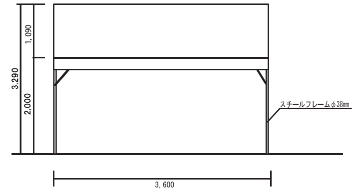
側面図
