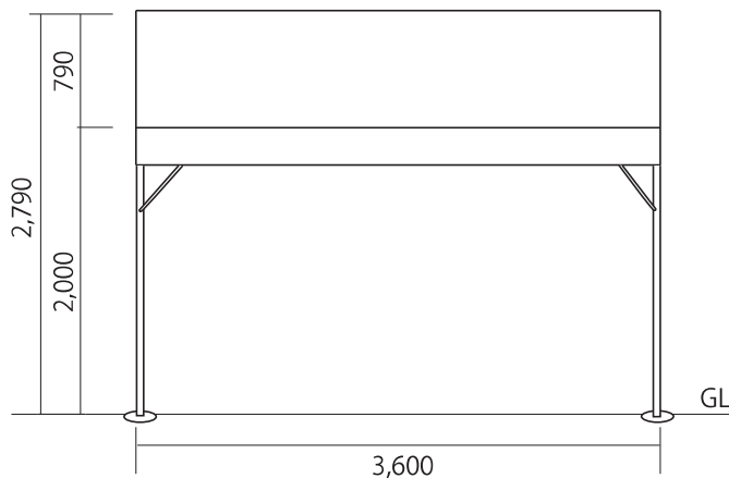
側面図
