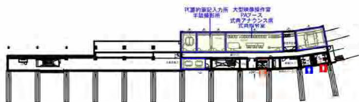
5階 平面図
